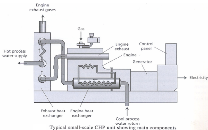
شکل ۴-۶- نوعی سیستم تولید مشترک برق و حرارت که مؤلفه‌های اصلی را نشان می‌دهد
