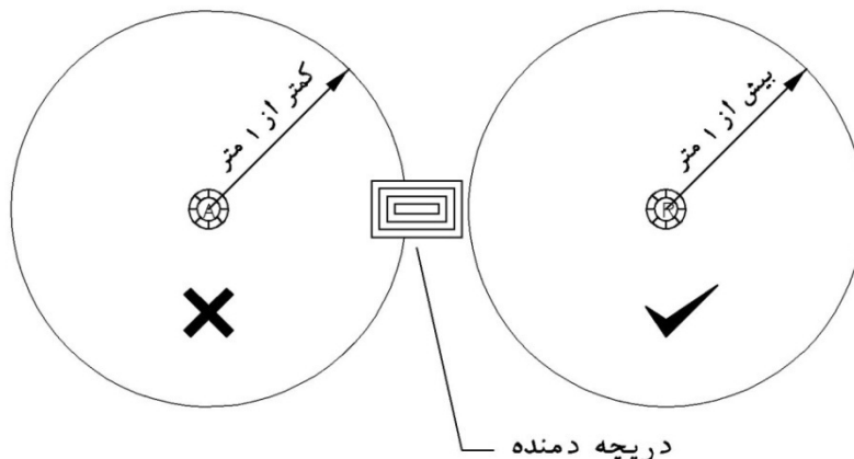
شکل ۳-۴-۱-۵- حداقل فاصله کاشف از دمنده های سقفی
