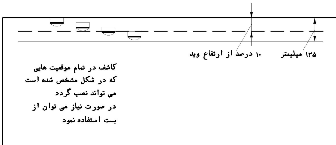
شکل ۱۲-۱-۴-۳- نصب کاشف در محدوده فوقانی وید
