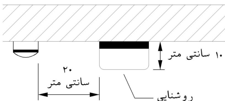
شکل ۱۳-۱-۴-۳- فاصله کاشف از سیستم روشنایی
