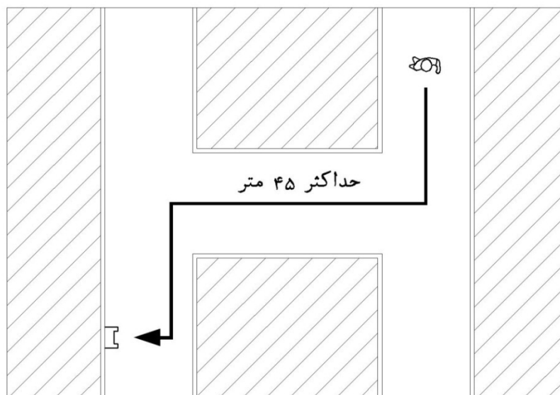
شکل ۳-۳-۴- حداکثر فاصله پیمایش تا شستی
